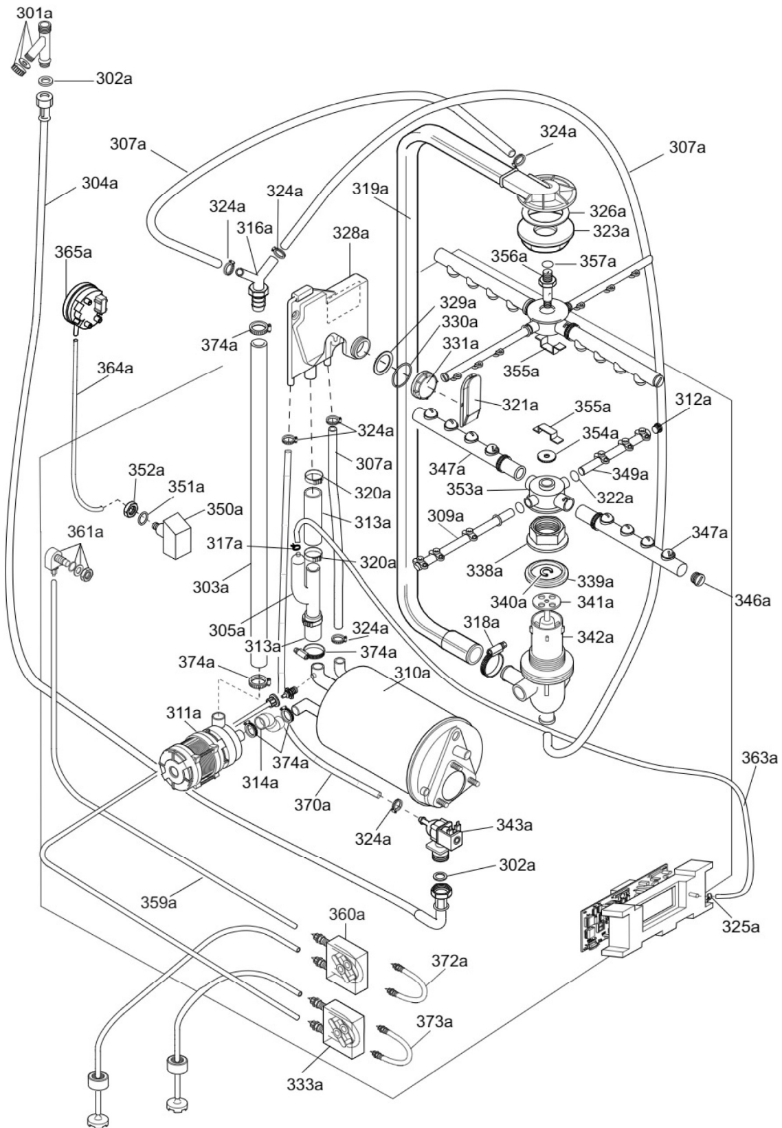
iii. 595665K00_p4B Circuito idraulico atmosferico / Atmospheric plumbing circuit
